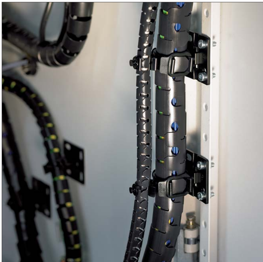
Kábelek és vezetékek védelme és rögzítése a Helawrap tartozékokkal ipari környezetben, mint például kapcsolószekrényekben.
