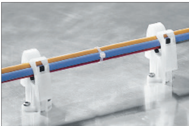
线束固定夹 HH20。
