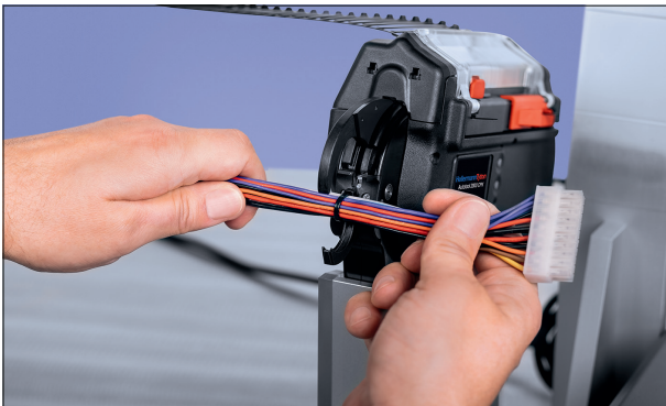
CPK悬空工作台工具应用
