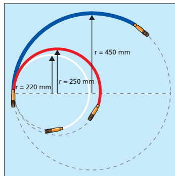
Oversigt over bøjningsradier
