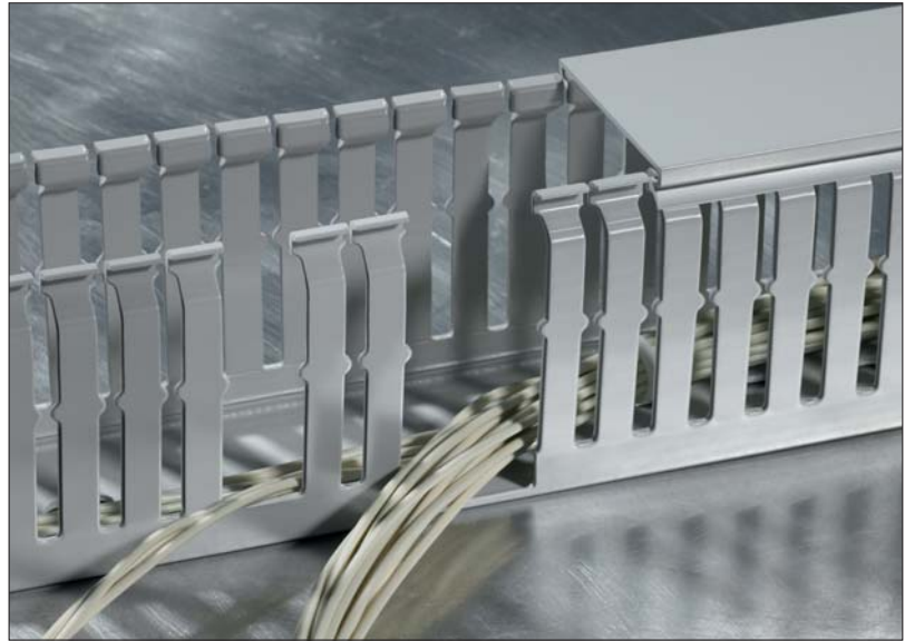
Verdrahtungskanal HTWD-HF.
