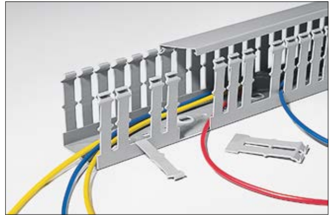
A HTWD-PW kábelcsatornák széles reteszekkel és résekkel rendelkeznek a nagy átmérőjű huzalok számára.
