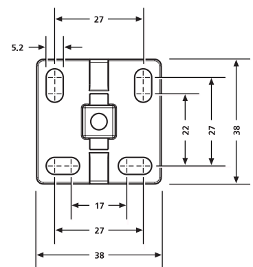
Helawrap HWBase/HWBaseA
