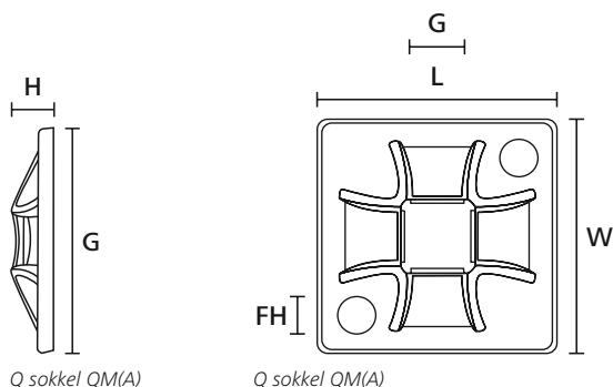
Q sokkel QM(A)
