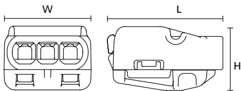
HelaCon genoplukkelig samlemuffe (forfra).
