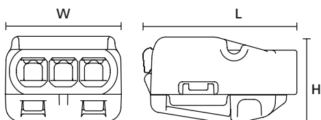
HelaCon öppningsbar frontvy.
