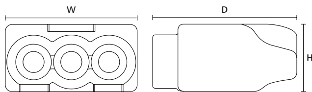
HelaCon Plus Mini framifrån
