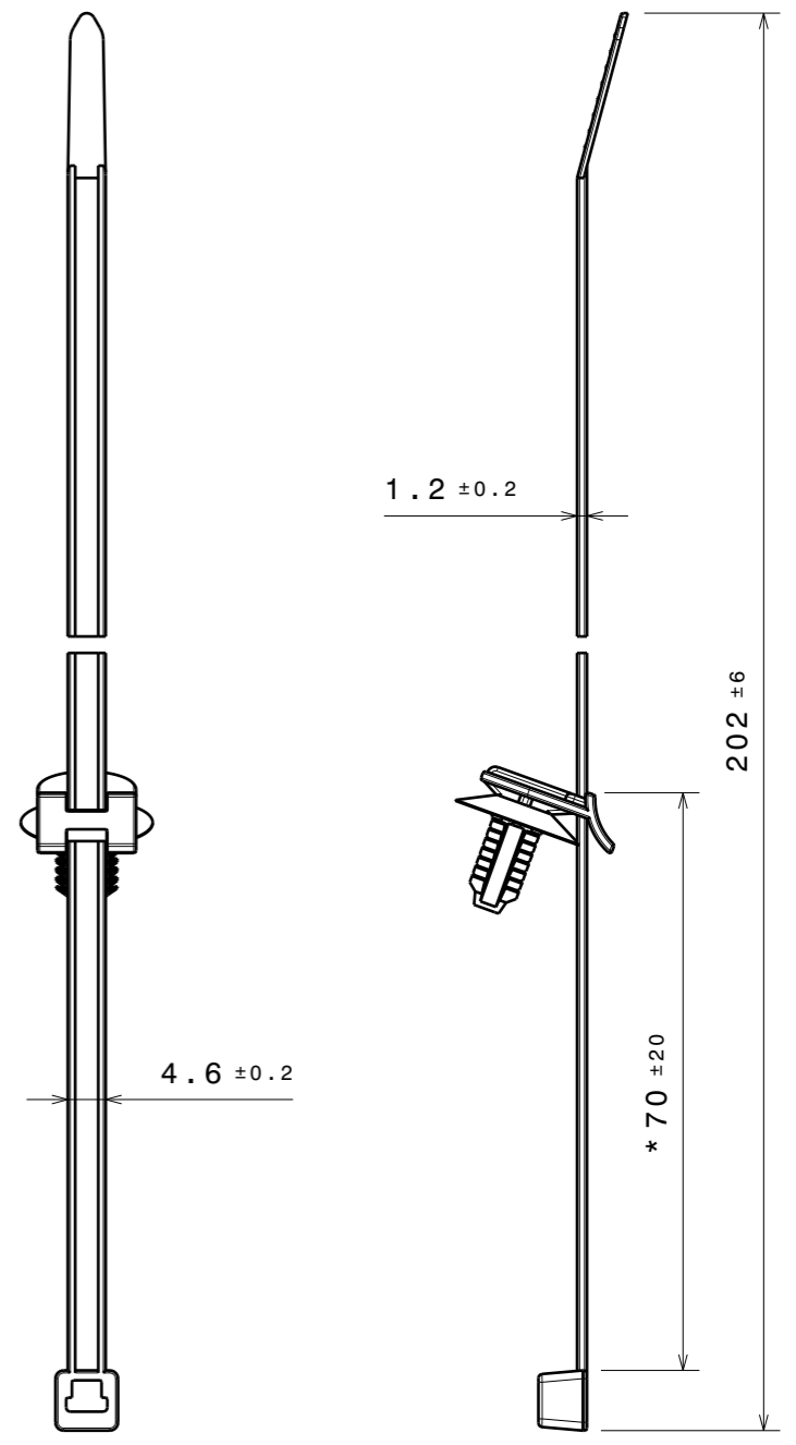
Agrafe livrée assemblée avec collier de serrage T50R PA46 Clip delivered assembled with cable tie T50R PA46
