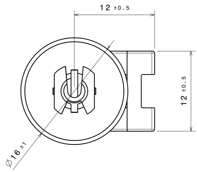
Vue de l'agrafe seule Clip alone View
