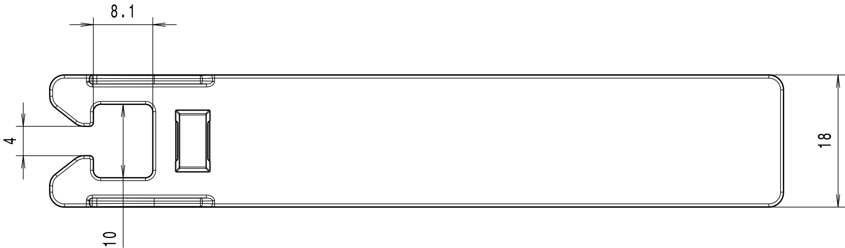
Aufnahme fuer Kabelbinder/ Retainer for cable tie (4.9 x 1.6)
