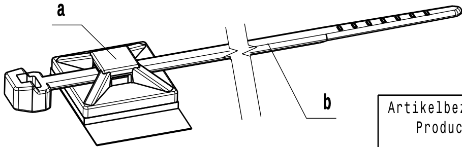
Montagebeispiel / Assembly example 2:1
