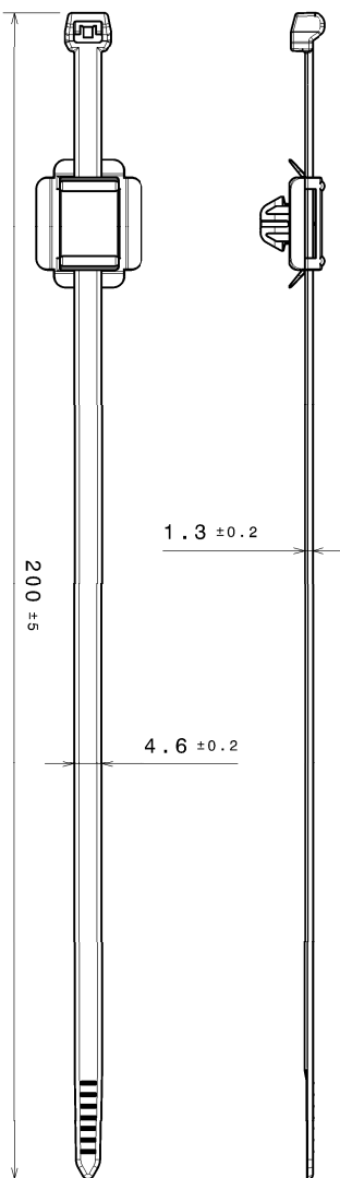
Assemblage avec collier T50ROSS Pour câblage Ø4 à 50mm maxi
