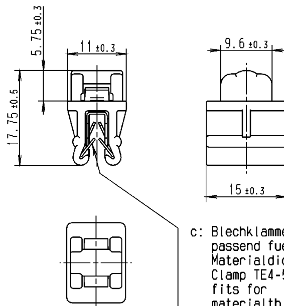
Sockel EC9/ socket EC9
