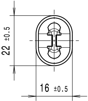
Ansicht ohne Dichtung/ View without seal
