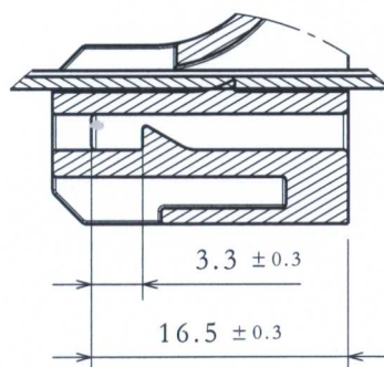
详图B 缩放: 2:1
