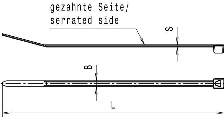
Lieferzustand / Delivery Condition Kabelbinder T... / Fixing tie T... 1:1
