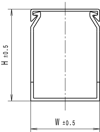
Montagezustand mit Deckel/ Assembled with cover
