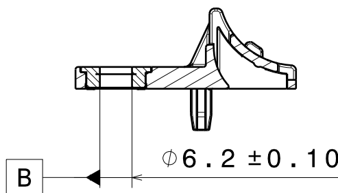
Section view A-A Scale: 1:1
