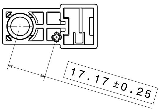
Bottom view Scale: 1:1
