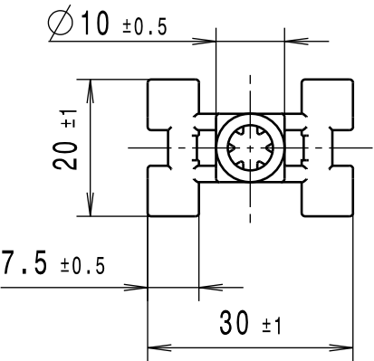
Ansicht ohne Kabelbinder/ View without cable tie
