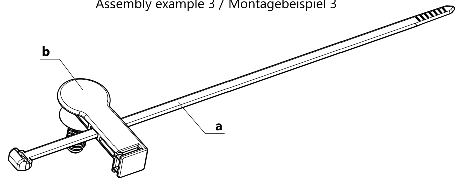
Assembly example 3 / Montagebeispiel 3
