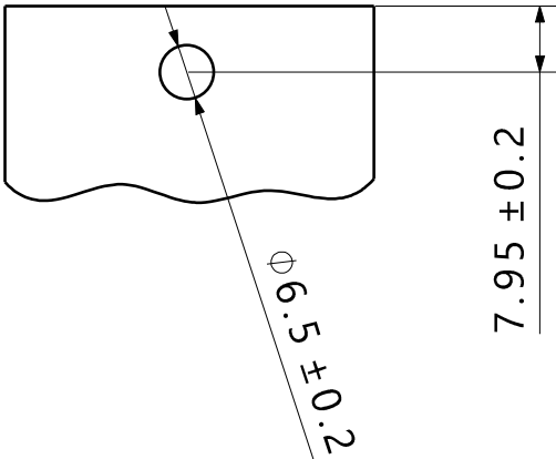
Hole pattern/ Lochbild
