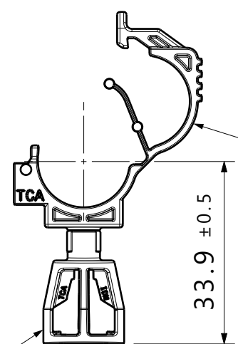
Stud mount
