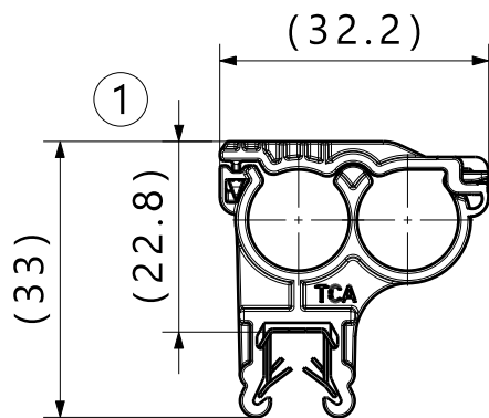
closed condition / geschlossener Zustand 1:1
