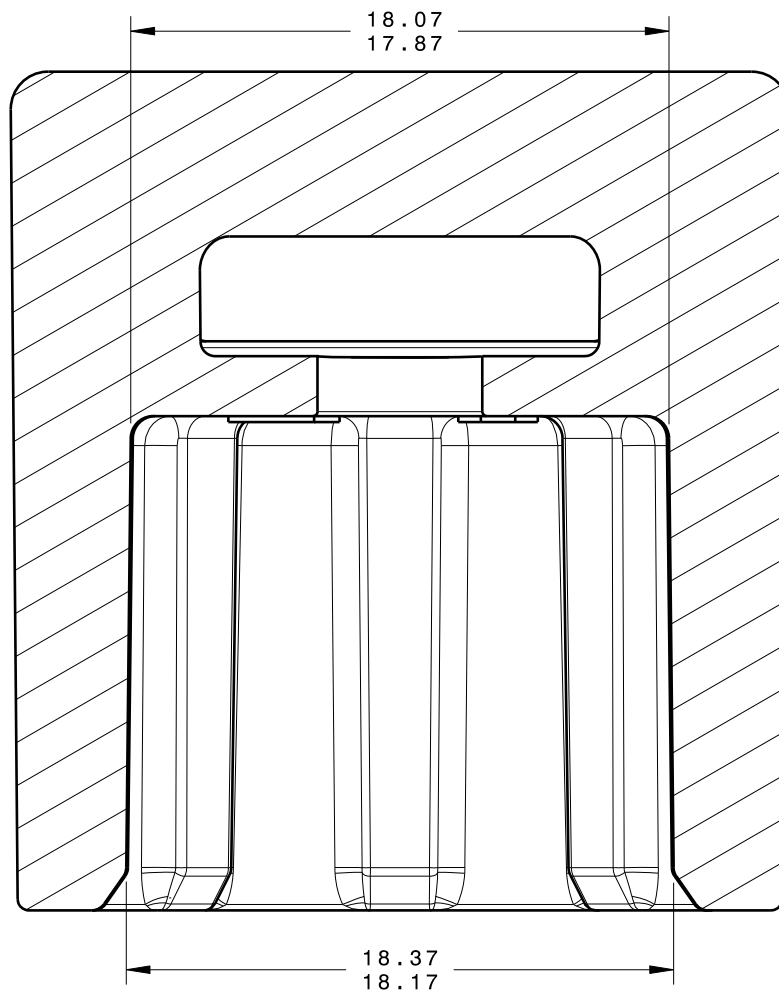
Section view A-A Scale: 4:1
