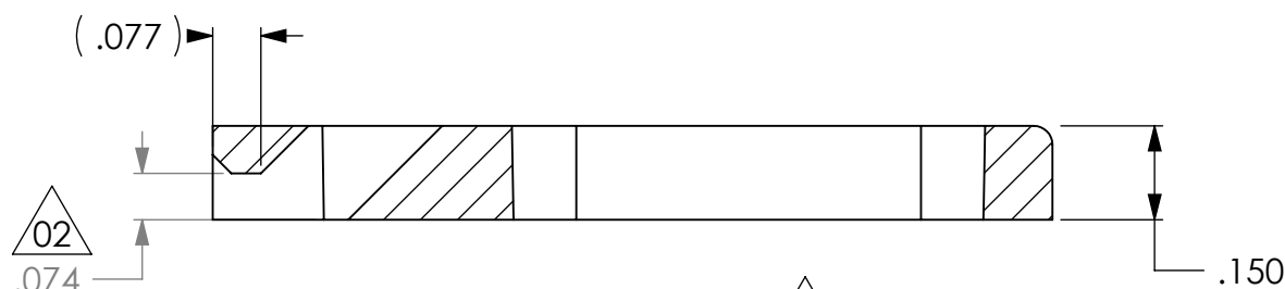
SECTION A-A
