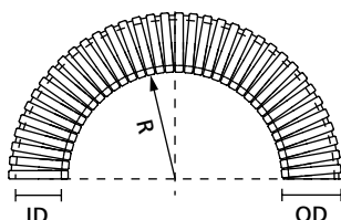
IWS non-metallic conduit
