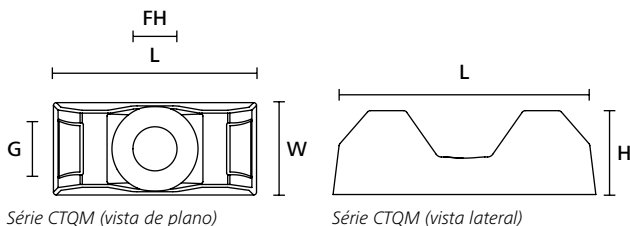
Série CTQM (vista de plano)
