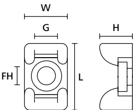
KR6G5, KR8G5 e CTM (vista de plano)
