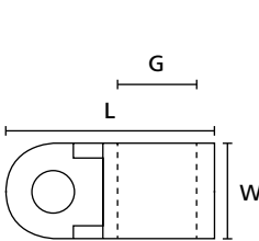
Bases TY3, TY8 (vista de plano)
