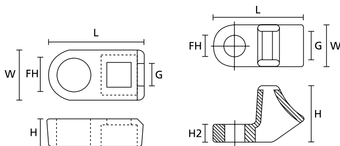
Bases de abraçadeiras FH (vista de plano e lateral)
