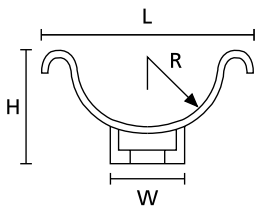
Abraçadeira berço (vista frontal)
