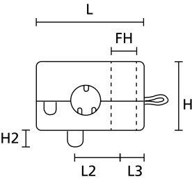
Klam-Klip (vista lateral)
