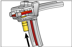
A cabeça destravada de uma abraçadeira KR.
