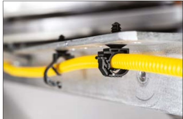
Os clips de travamento da série LOC oferecem agrupamento fácil e rápido de tubos lisos ou corrugados.
