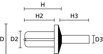
Rebite de plástico TY3P1 / 8P1
