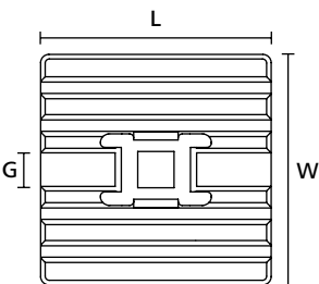
Base adesiva flexível FMB4APT-A (vista de plano)
