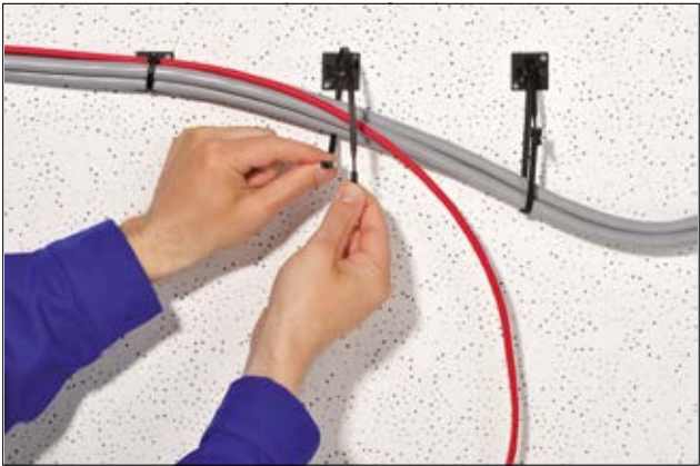
As abraçadeiras Q podem ser usadas para instalação temporária e final de cabos.
