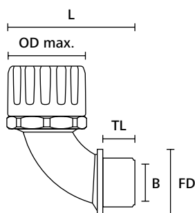
Bucim HelaGuard, 90 ° com rosca interna fixa
