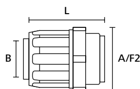
Bucim FlexiGuard, reto com rosca giratória
