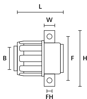
Bucim FlexiGuard, reto com suporte
