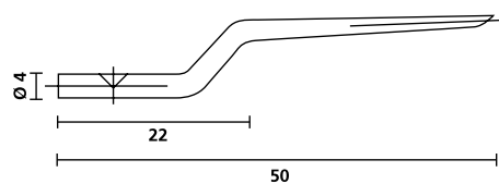
Bicos de substituição NA1K/3
