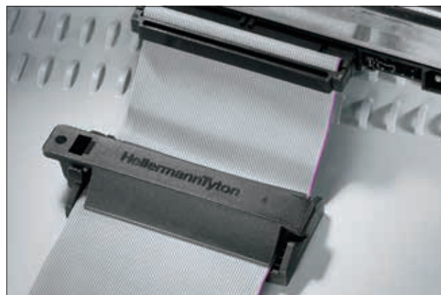
Clip pour câbles plats de la série FKH, en application.
