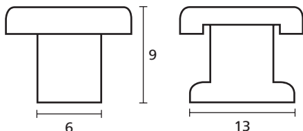
HTWD-TL Mount
