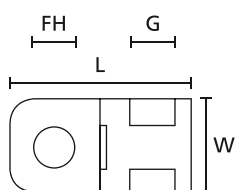
CTAM-serie (bovenaanzicht)
