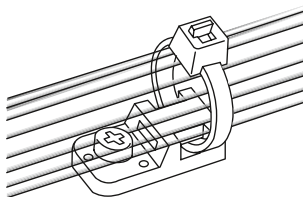
CTAM1/CTAM2 bevestigingszadels
