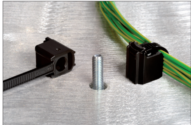
LFC165-2 - max. 35,0 mm nipun halkaisijoille.
