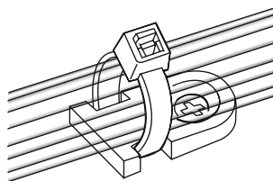
Schéma d'une embase série MB, en application
