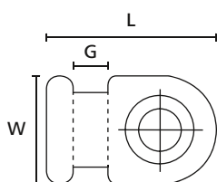
Embase série MB (vue du dessus)
